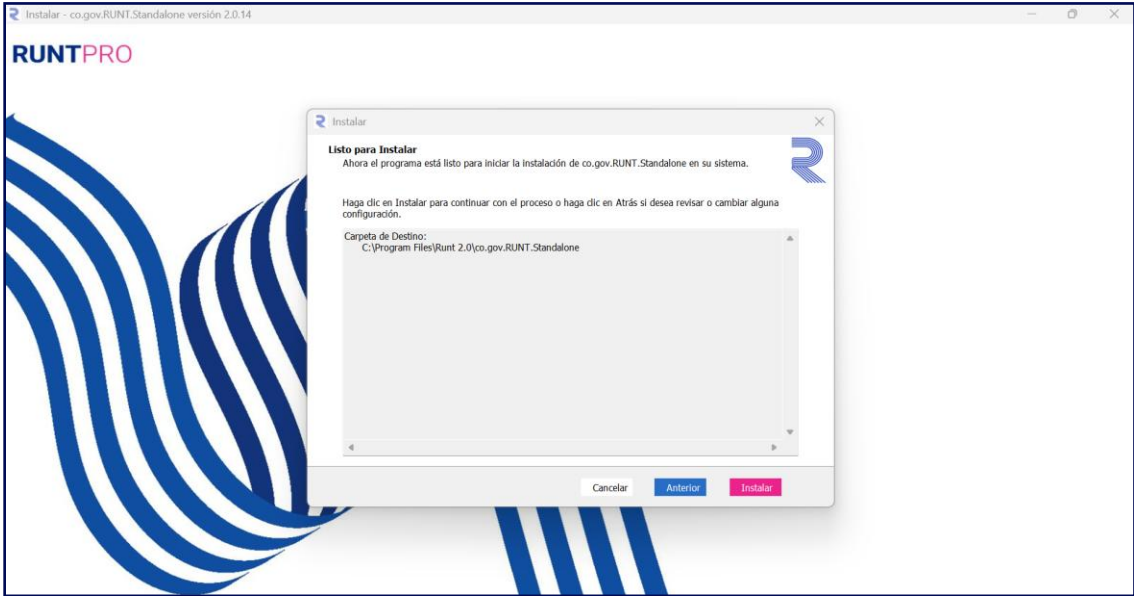
Imagen 52 – Opción instalar
