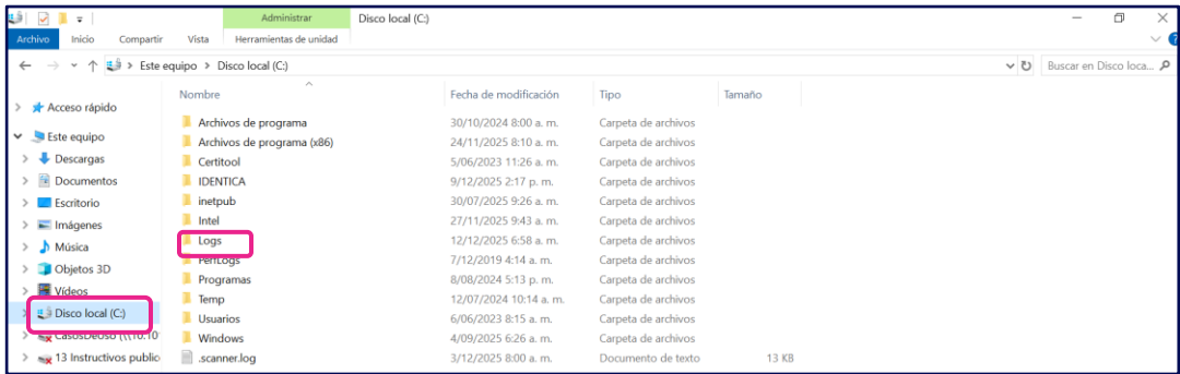
Imagen 58 – Ruta logs
