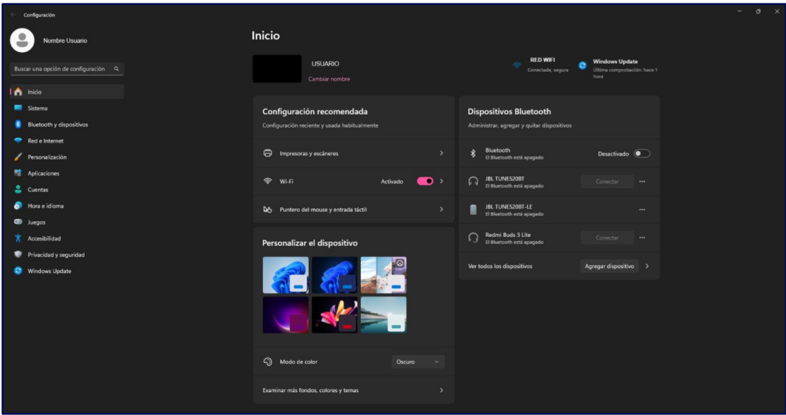
Imagen 2 – Configuración Windows 11
