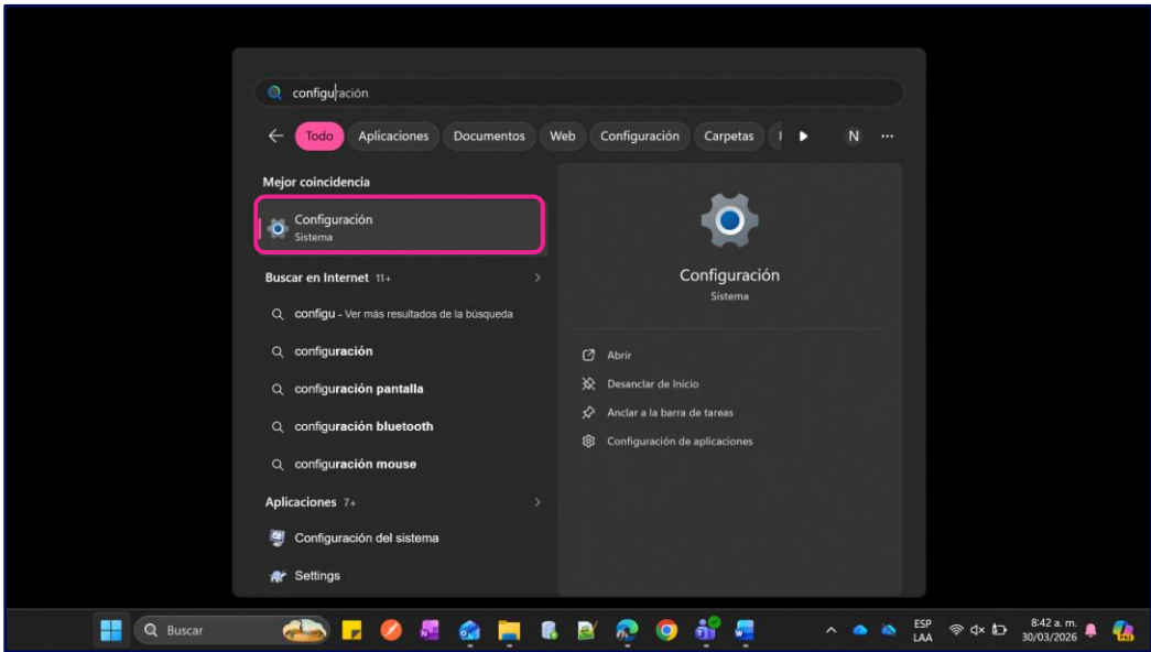
Imagen 1 – Escritorio Windows 11
