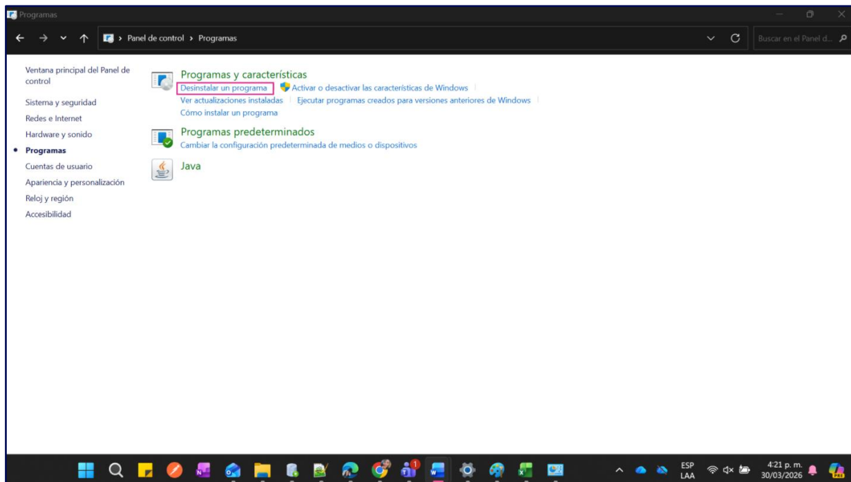
Imagen 12 – Desinstalar programas
