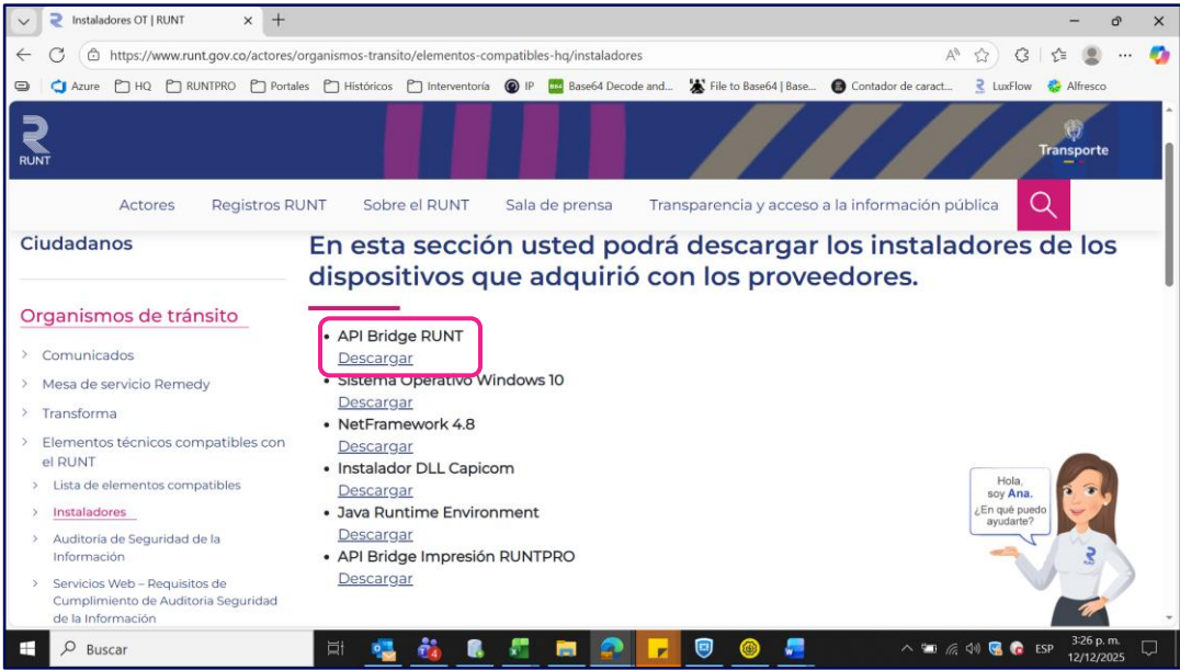
Imagen 47 – Descargar Bridge
